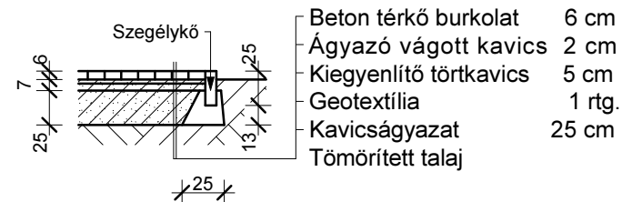
A-A metszet M 1:50
